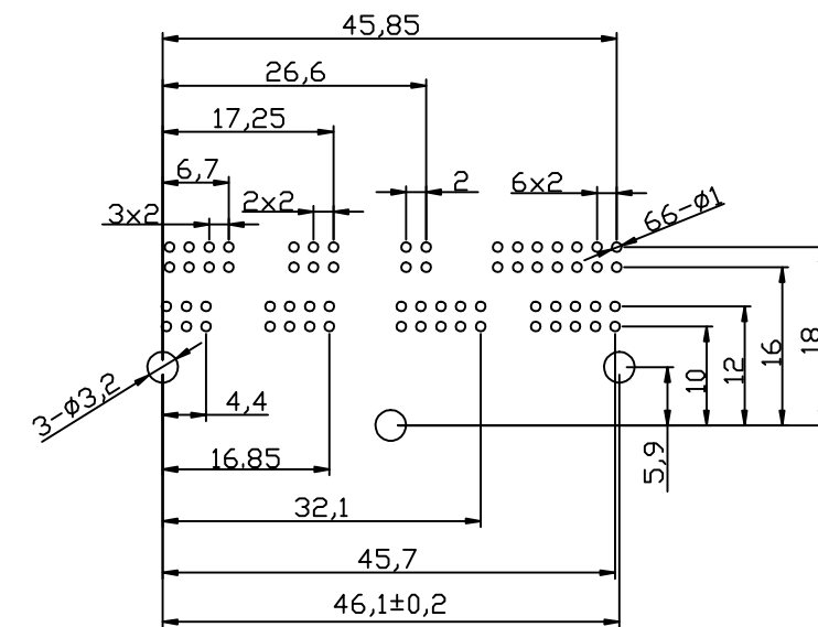
印制板安装开孔图
